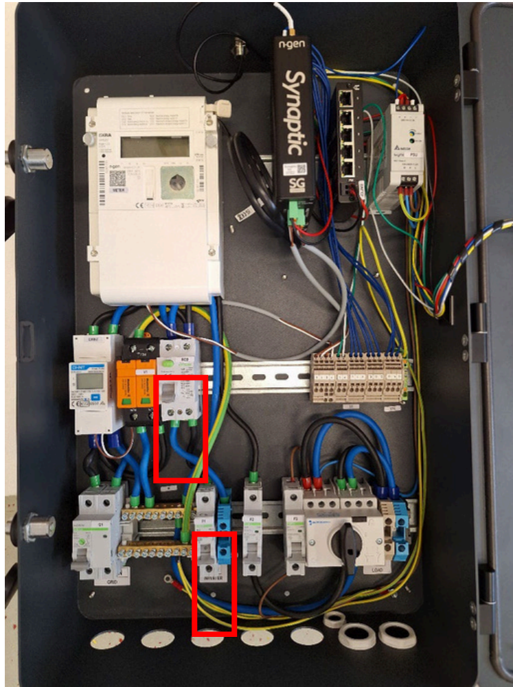
Slika 20: Isključivanje osigurača invertera i RCD-a
