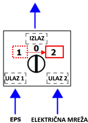
Slika 29: Preklopni prekidač
