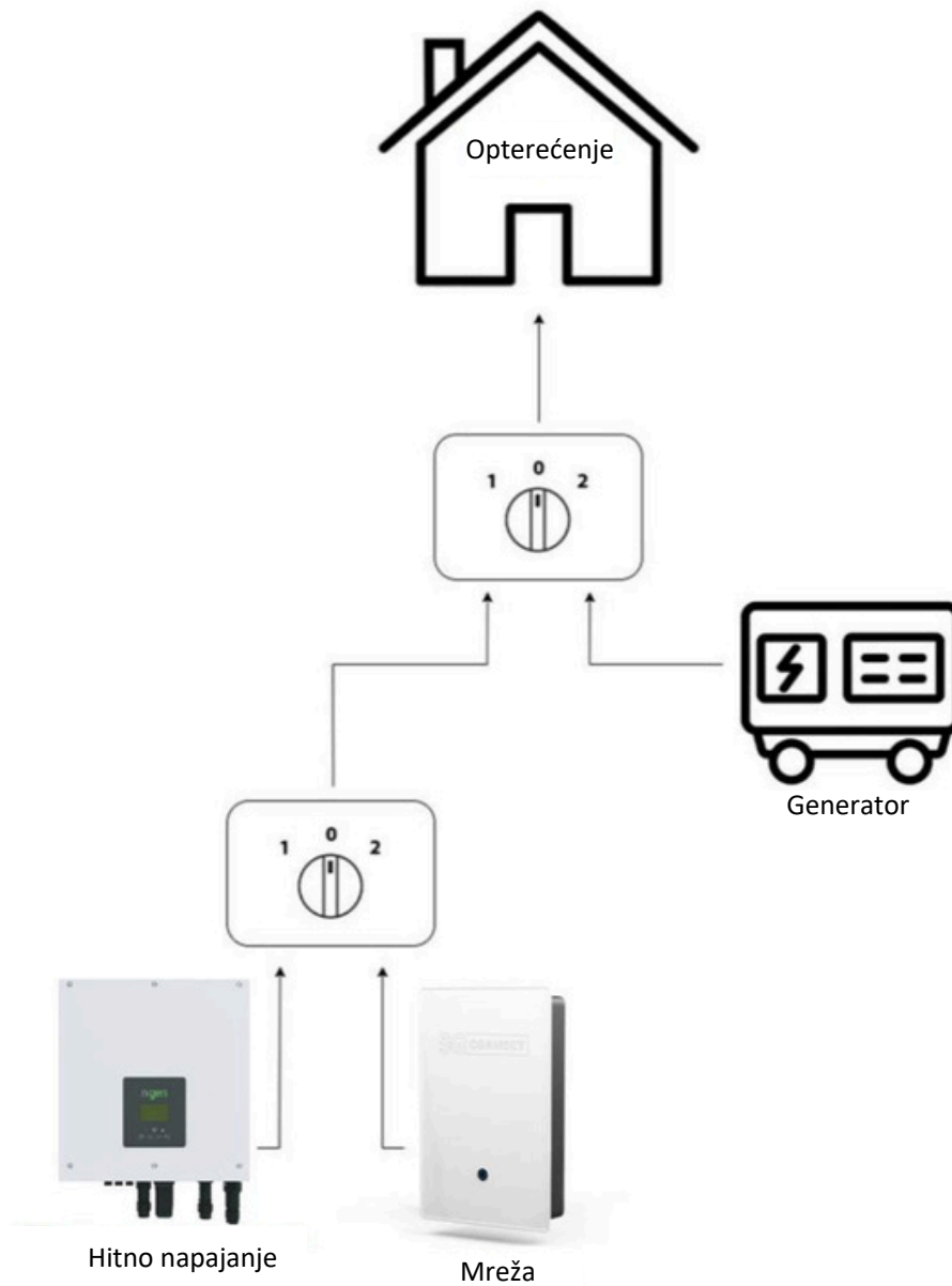
Slika 12: Spajanje agregata
