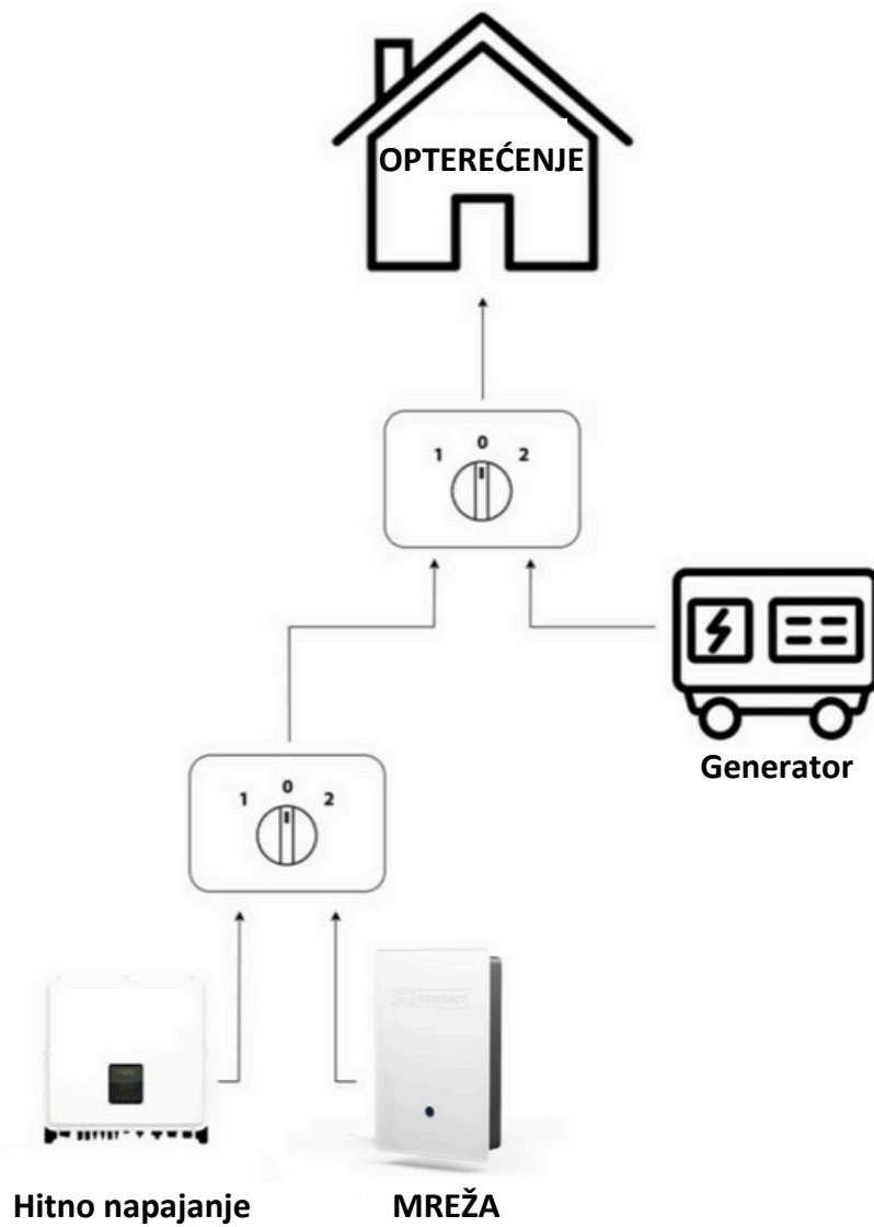
Slika 12: Spajanje agregata
