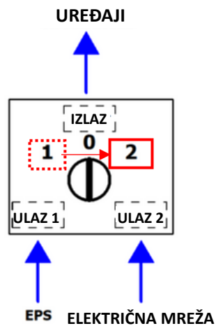
Slika 29: Preklopni prekidač
