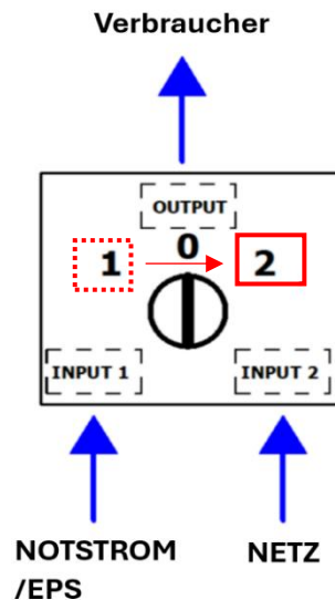
Abbildung 29: Netzumschalter
